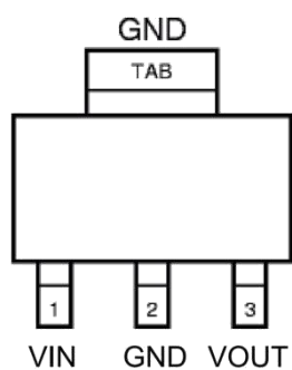
SOT-223
